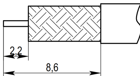
Рисунок 2 Пример разделки кабеля
